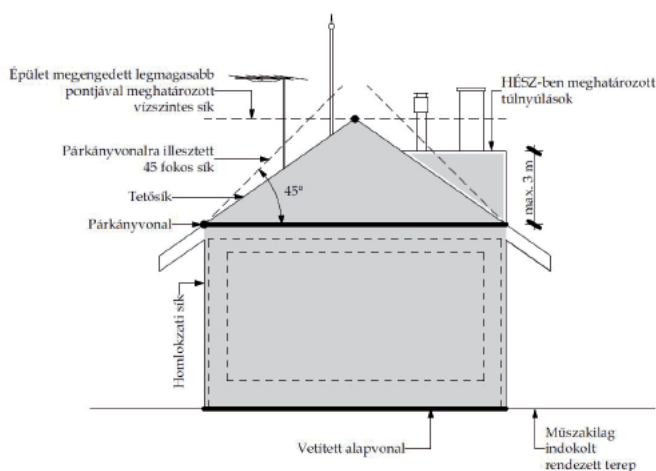
SÍK TEREPEEN, MAGASTETŐS ÉPÜLET BEÉPÍTÉSI MAGASSÁGA
