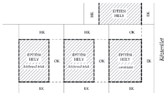
Közterület OLDALHATÁRON ÁLLÓ BEÉPÍTÉSI MÓD
