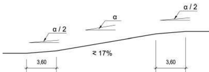
2. ábra: az álláshelyekhez vezető lejtő (közlekedési rámpa)
